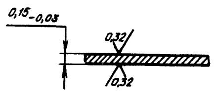
Ось пружин
